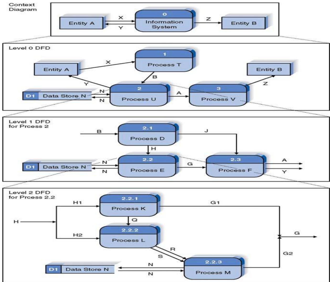
Gambar 8.3 Hirarki penyusunan DFD Keterangan :
