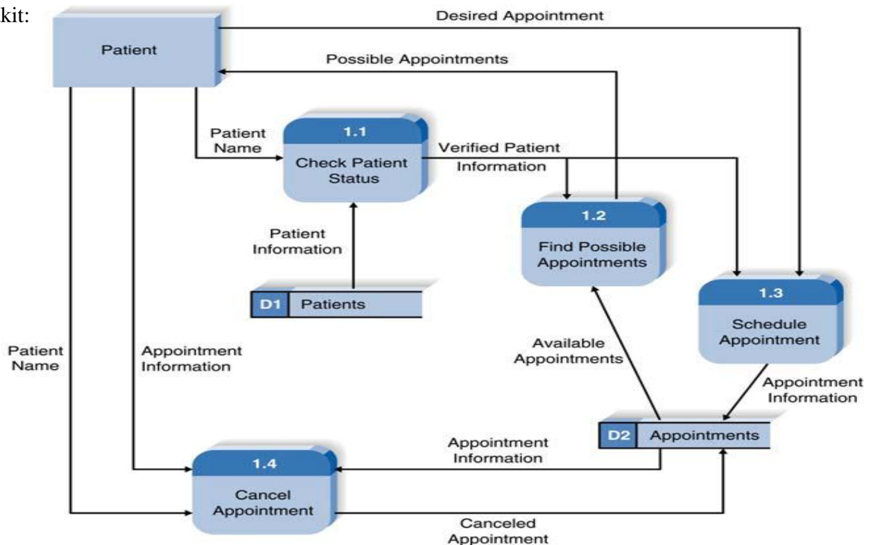
Gambar 8.1 DFD
