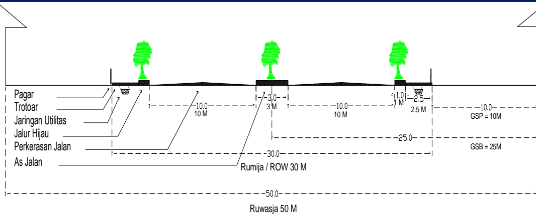
Penampang Jalan Arteri
