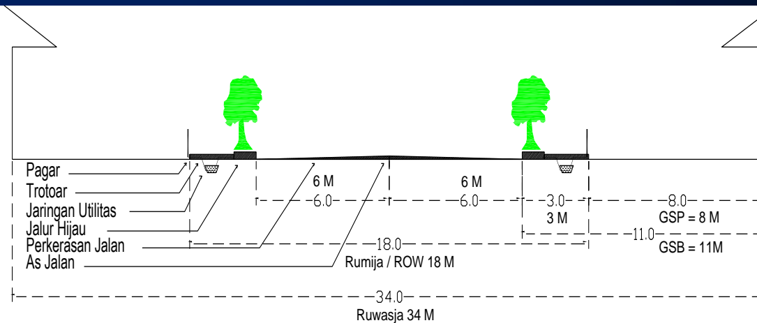
Penampang Jalan Kolektor
